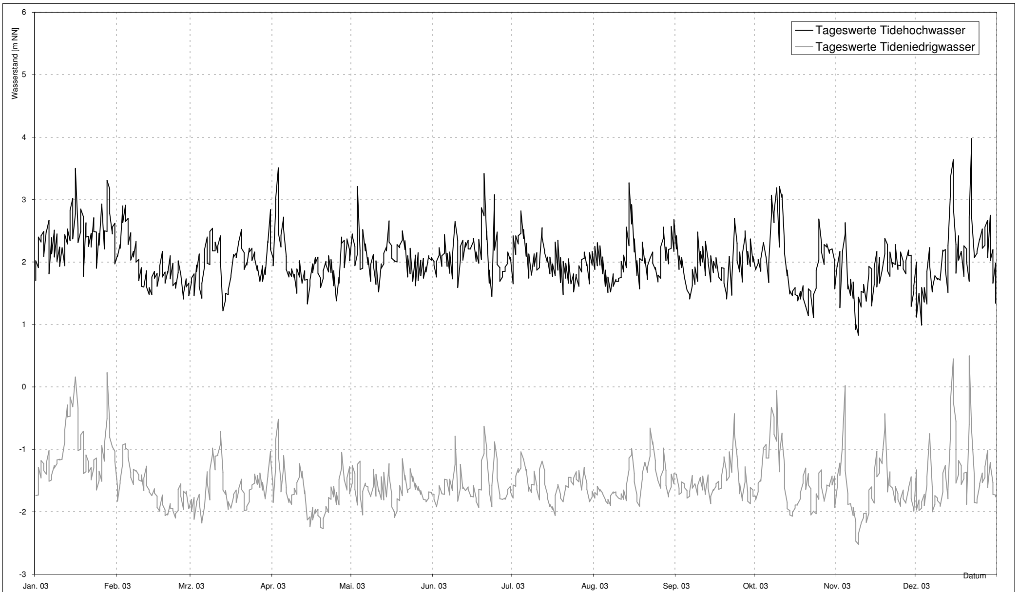
Abb. I-2.2: Tageswerte der Tidewasserstände am Elbpegel St. Pauli vom 01.01.2003 bis 31.12.2003
