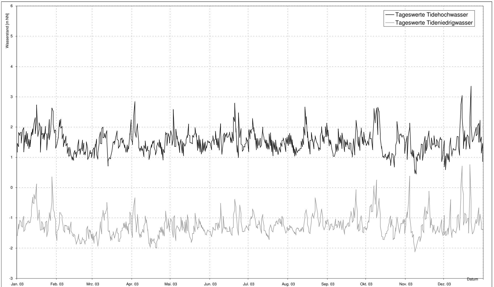
Abb. I-2.1: Tageswerte der Tidewasserstände am Elbpegel Glückstadt vom 01.01.2003 bis 31.12.2003
