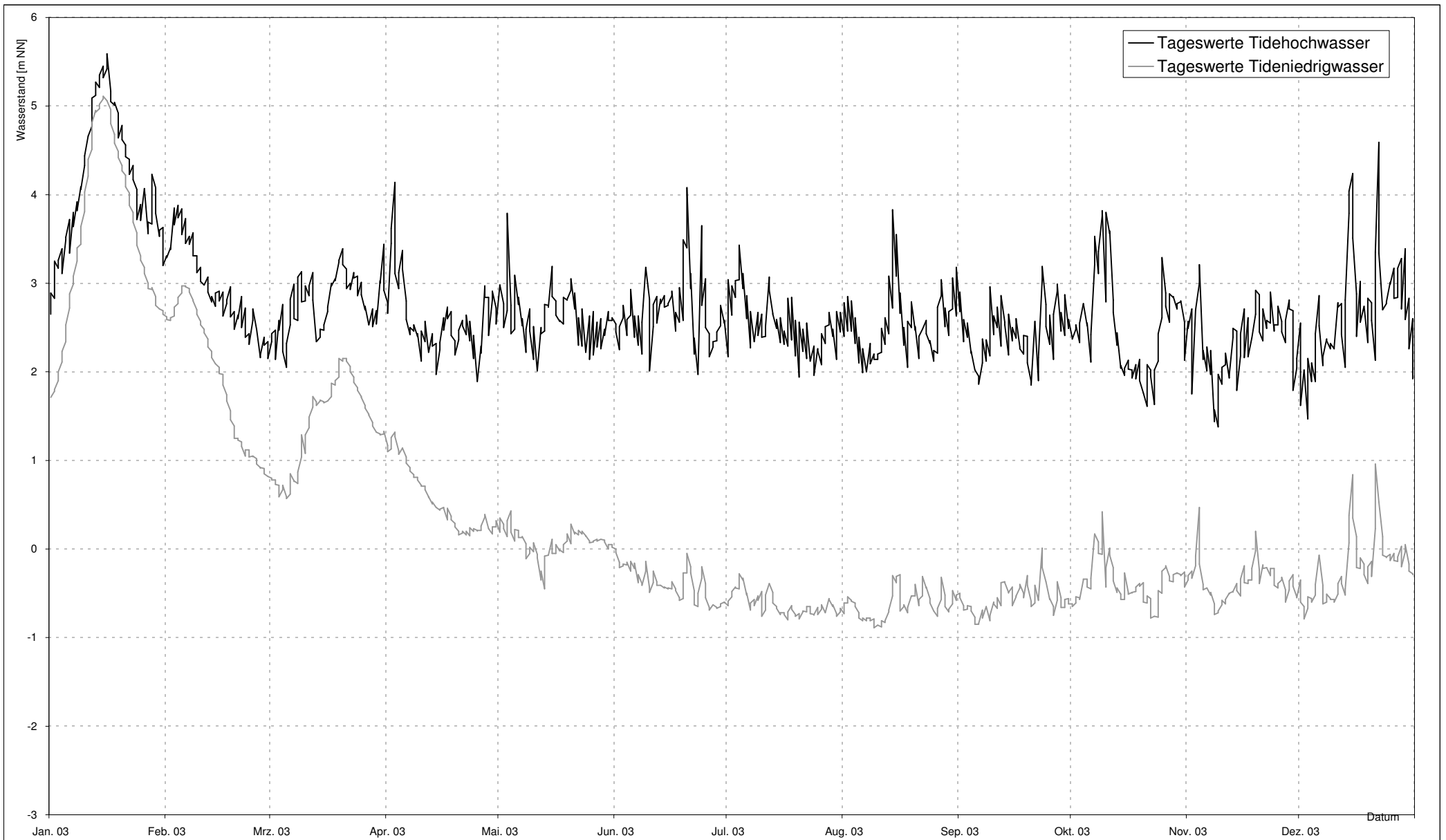
Abb. I-2.3: Tageswerte der Tidewasserstände am Elbpegel Geesthacht vom 01.01.2003 bis 31.12.2003
